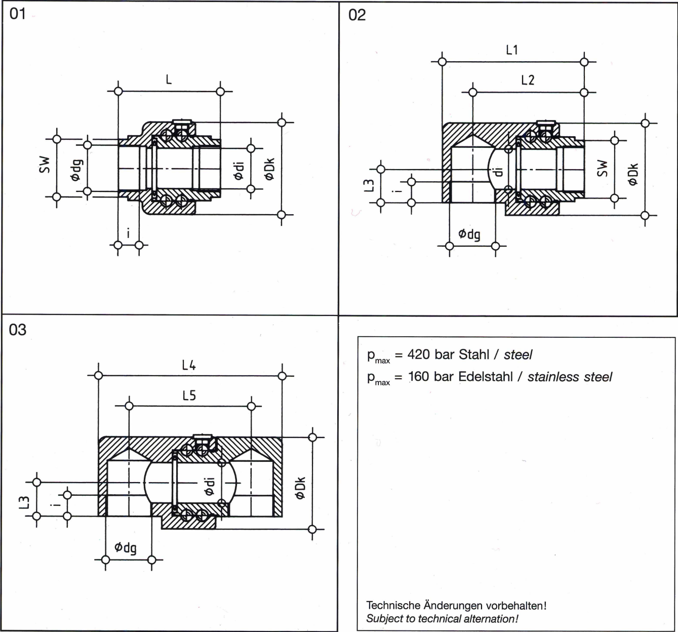
Abmessungen (mm) Stahl und Edelstahl Dimensions (mm) steel and stainless steel Gewichte (kg) Weights (kg)
